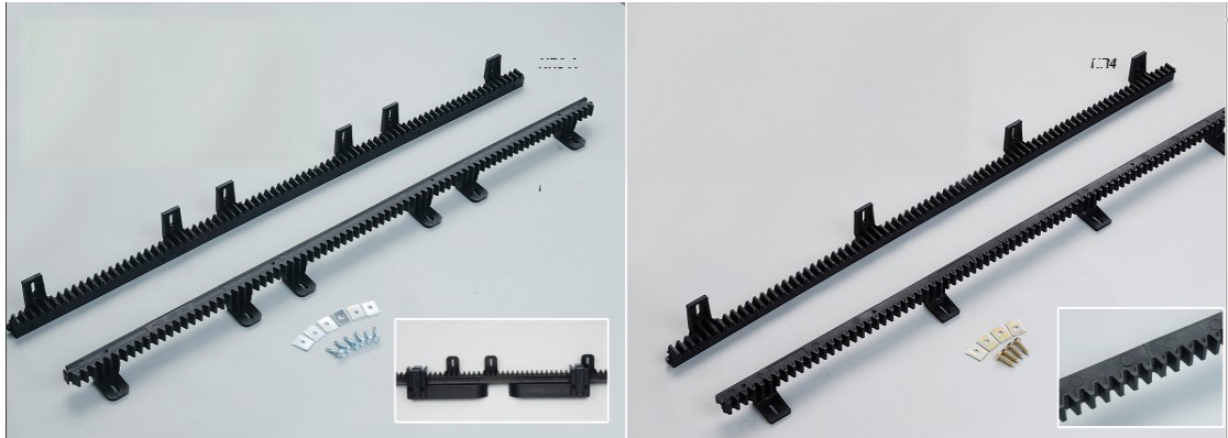
Nylon gear racks /Cremallera Nylon /Нейлон стойки передач/cremaillere en Nylon/ رفوف والعتاد النايلون
